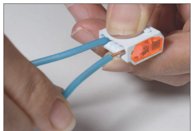
החדרה חלקית
