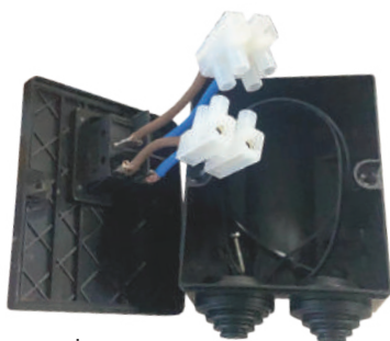
חיווט מלא
