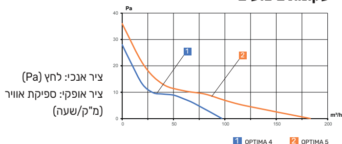
עקומת ביצועים
